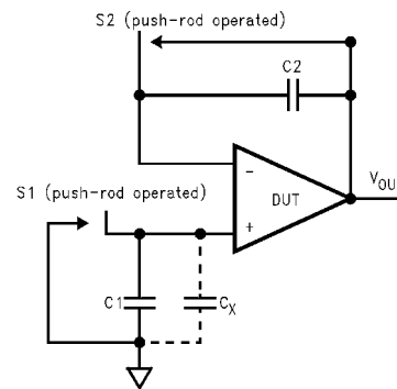
FIGURE 8. 入力バイアス電流試験の簡略回路
