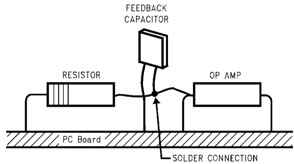
FIGURE 7. 空中結線
